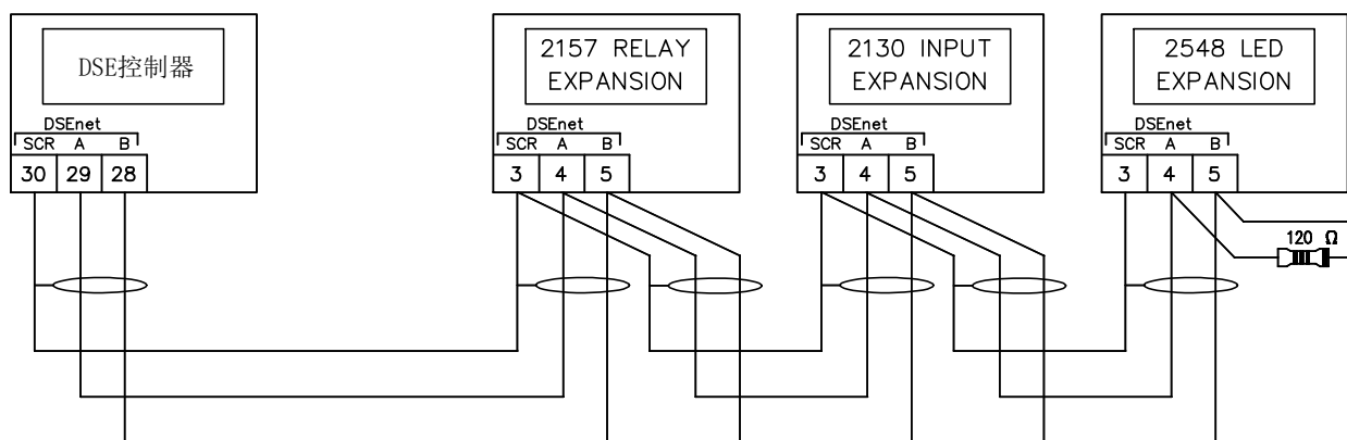
扩展模块与控制器通讯接线图
