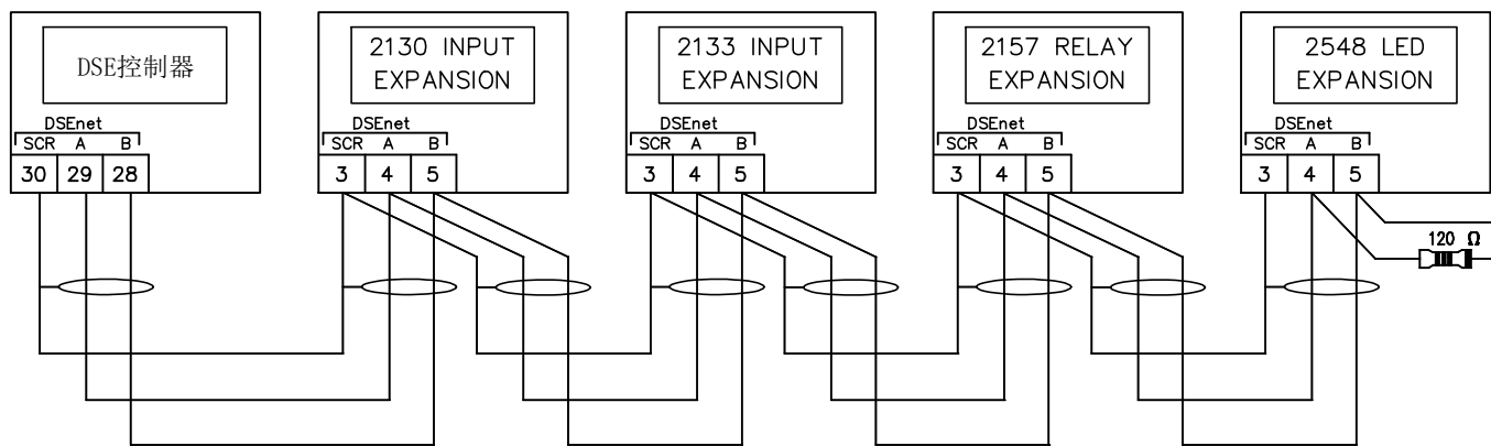
扩展模块与控制器通讯接线图
