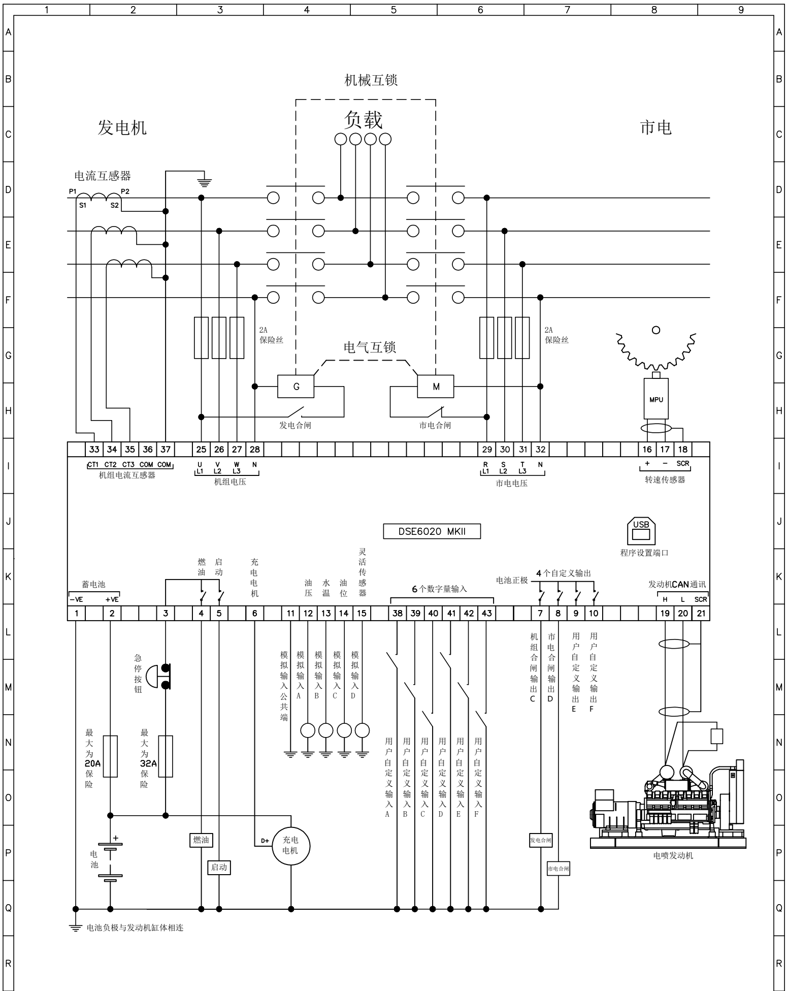
DSE6020 MKII 典型接线图 图纸编号: 版本 1 页码 1/1
